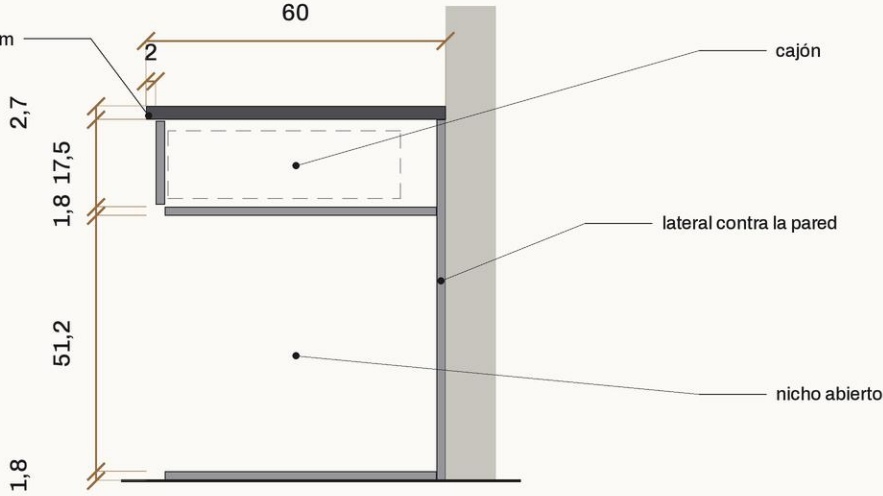
CORTE POR LA CAJONERA
